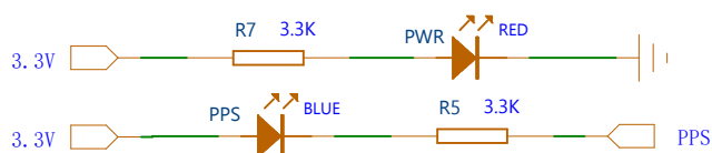
LED指示电路
